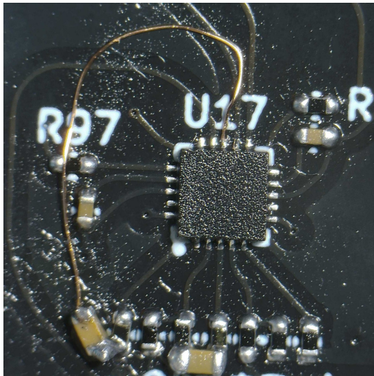
(a) Firul ce leaga unul dintre LDO-uri de un condensator.
