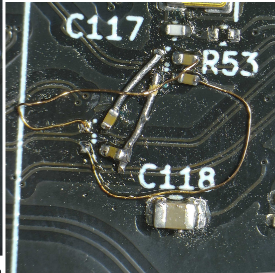
(b) Repararea liniilor USB prin lipirea unor fire.
